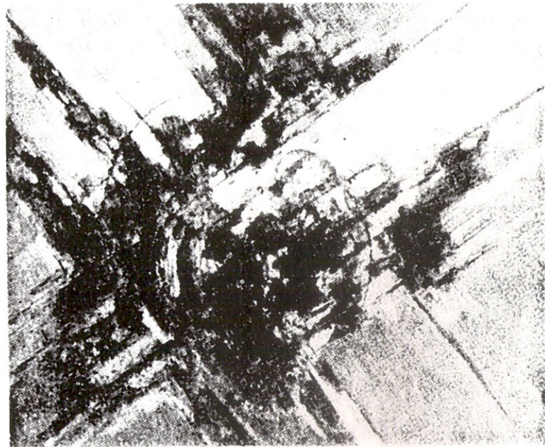
שישקריה פרדינאנדו - דינמיקה גרעינית
